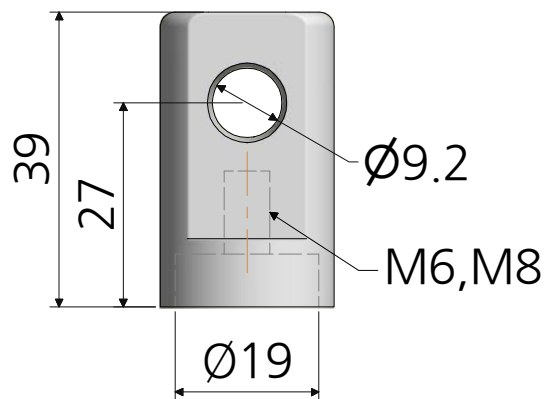
다대보고정대 - 39 RG6-39 : M6 RG8-39 : M8
