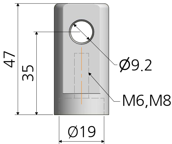
다대보고정대 - 47 RG6-47 : M6 RG8-47 : M8
