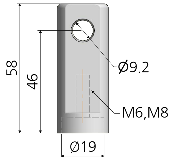
다대보고정대 - 58 RG6-58 : M6 RG8-58 : M8
