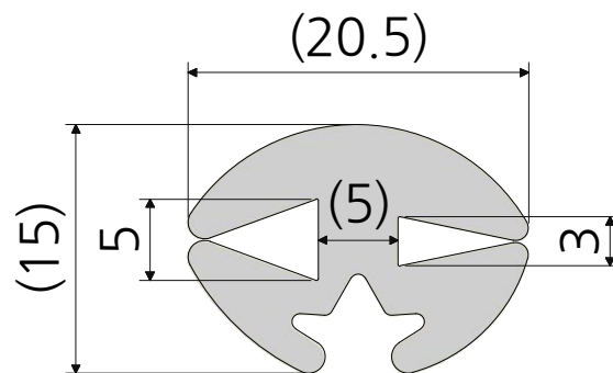
유리패킹 중 PK-G6-2
