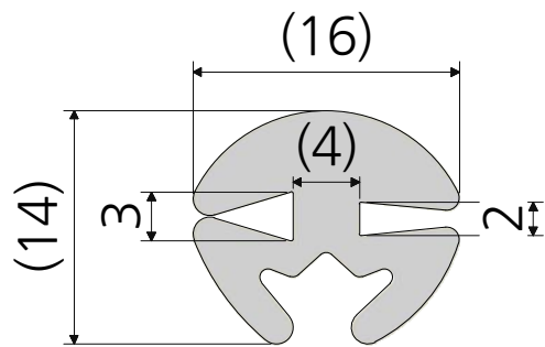
유리패킹 소 PK-G6-1
