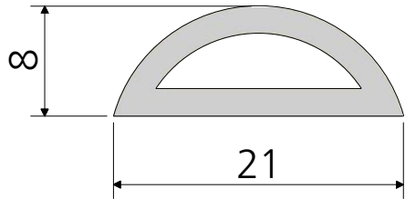
D형패킹 소 〈PK-D1-1〉
