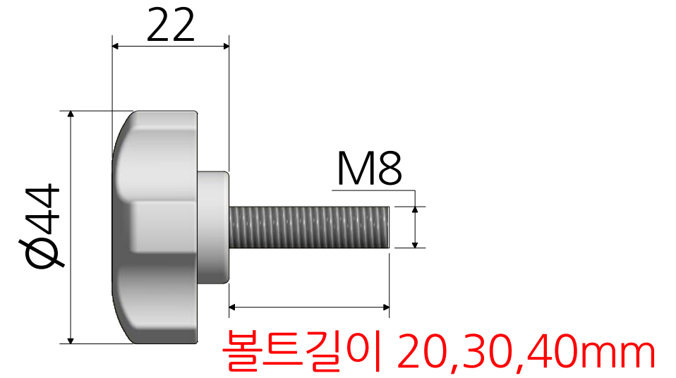
FKB-M8-볼트길이
