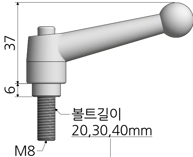
CLBS-C8-( 볼트길이 )
