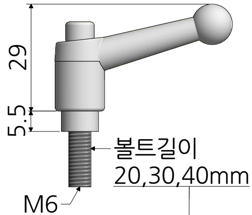
CLBS-C6-( 볼트길이 )
