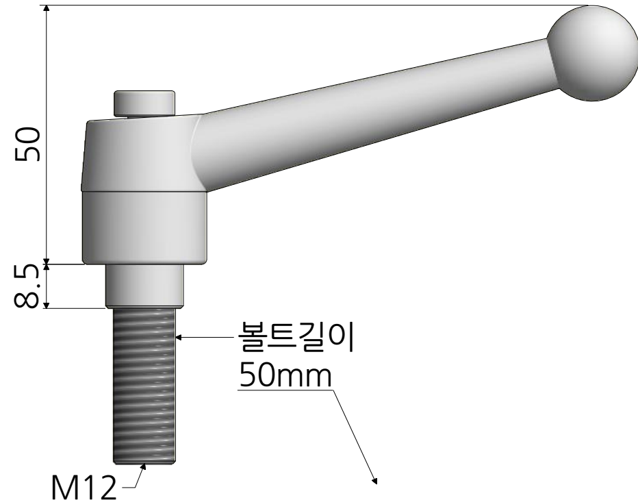
CLBS-C12-( 볼트길이 )
