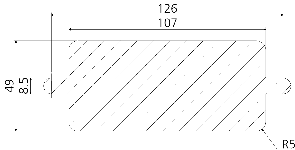
< 타공도 >
